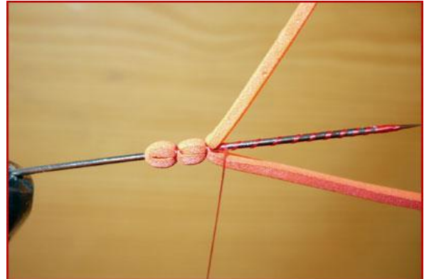
Etape 6 : emprisonner à nouveau la mousse (toujours 2 tours bien serrés) pour former la deuxième partie de l'abdomen puis remettre un tour de soie sous la mousse/sur l'aiguille.
