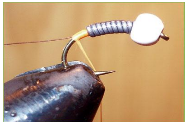
Etape 4 : fixer à la courbure un morceau de fil de cuivre fin.
